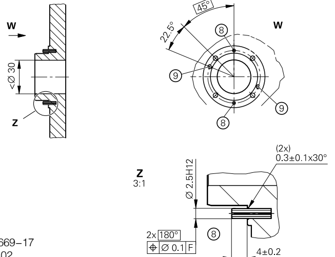
前端联轴器 带机械故障防护 (有关更多尺寸, 参见“无机机械故障防护”)
