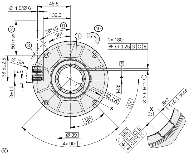
带环形螺母联轴器 无机机械故障防护
