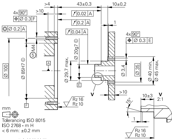
前端联轴器 无机机械故障防护
