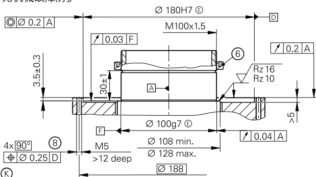
轴连接用环形螺母与棘轮 带机械故障防护 (有关更多尺寸, 参见“无机机械故障防护”)
