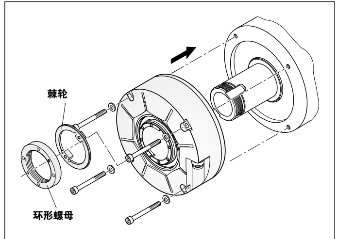
带环形螺母和棘轮的联轴器
