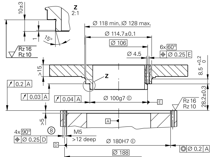
前端联轴器 带机械故障防护 (有关更多尺寸, 参见“无机机械故障防护”)
