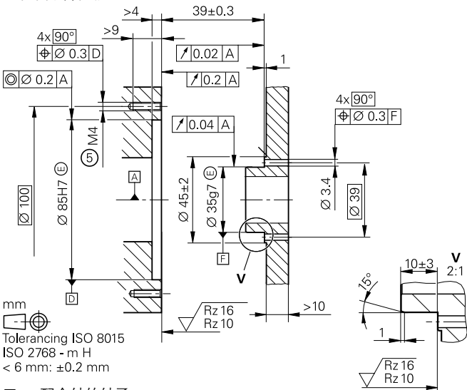
前端联轴器 无机机械故障防护
