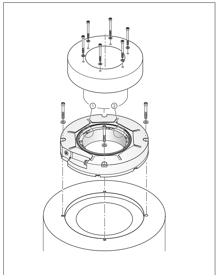
连接编码器与轴端面举例
