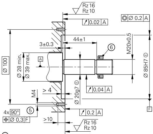
前端联轴器 无机机械故障防护
