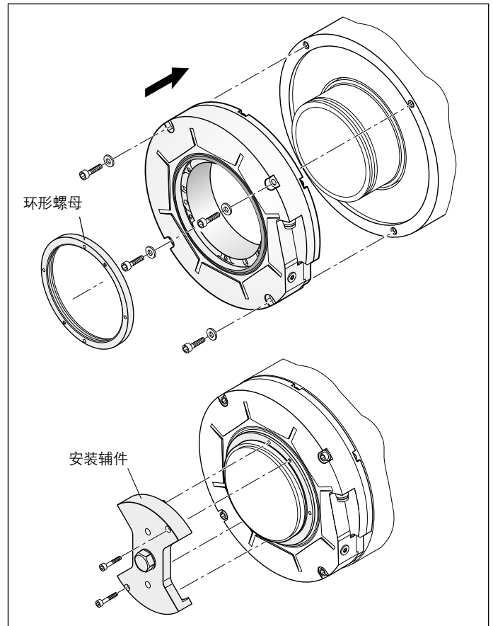
用环形螺母安装角度编码器
