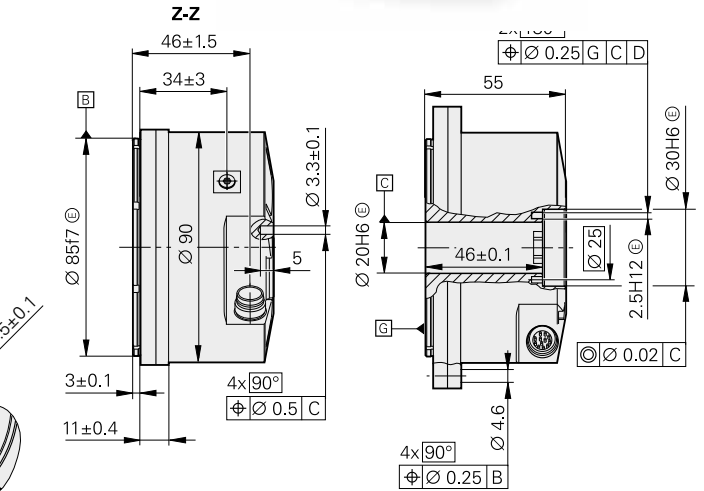
带环螺母和棘轮的联轴器 带机械故障防护 (有关更多尺寸, 参见“无机机械故障防护”)
