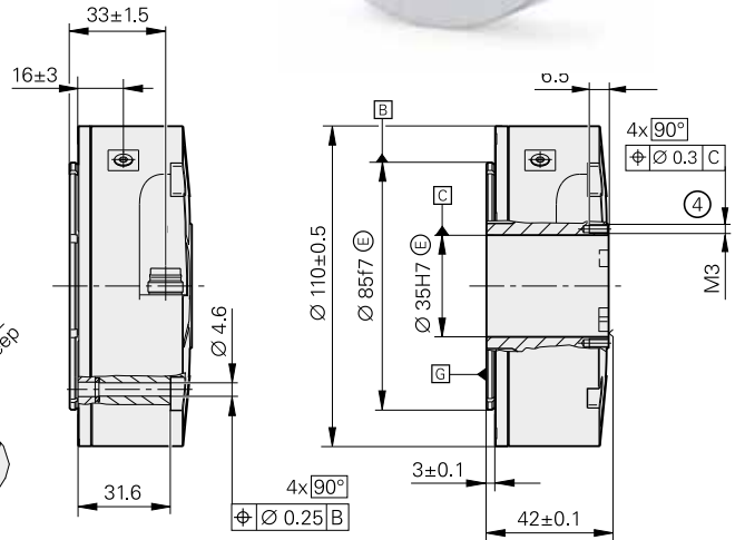
带环形螺母和棘轮的联轴器 带机械故障防护 (有关更多尺寸, 参见“无机机械故障防护”)
