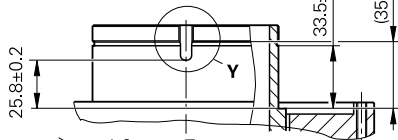
图示中无环形螺母和棘轮
