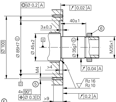
前端联轴器 无机机械故障防护
